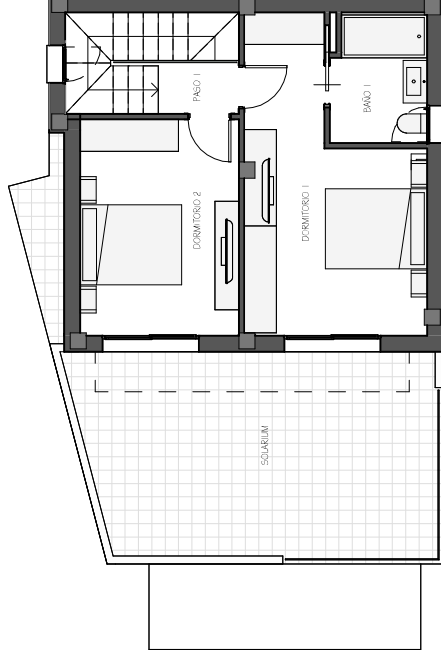
PLANTA 1
